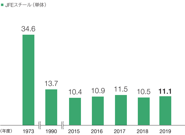
JFEスチールのNO x 排出量推移(百万Nm 3 )
